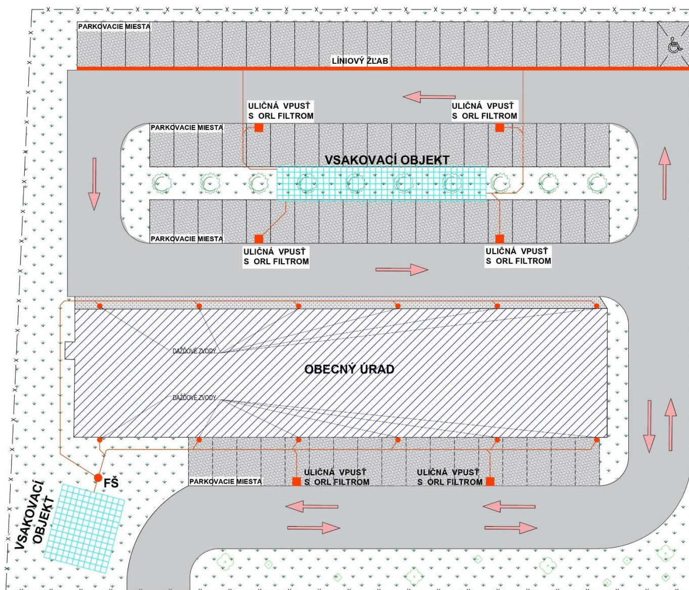
Situácia – Vzorové riešenie pre objekt obecného úradu
